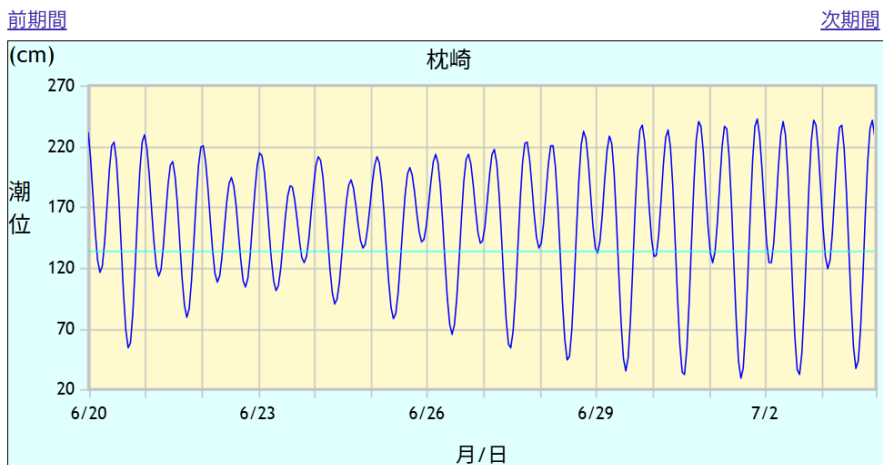
毎時潮位グラフ 枕崎 2026年6月20日～2026年7月3日の潮位予測
