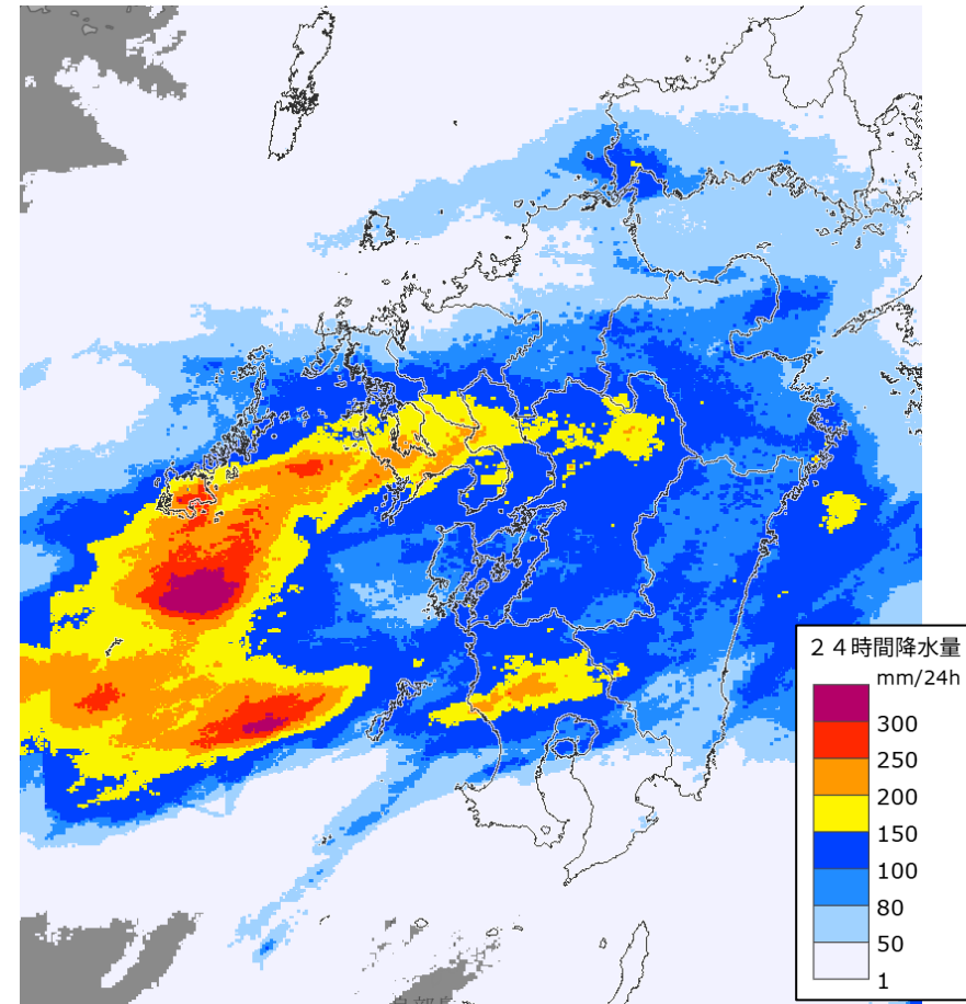
24時間解析雨量(24日12時)
