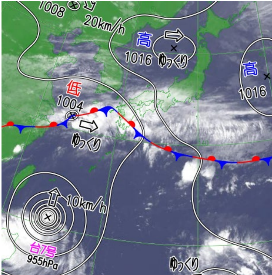
気象衛星画像と天気図(24日9時)
