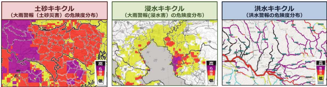
土砂・浸水・洪水キキクルの表示例
