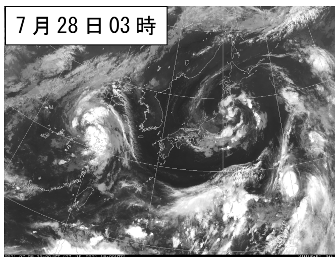
(3) 地上天気図及び気象衛星赤外面像 7月28日03時～29日15時：6時間毎
