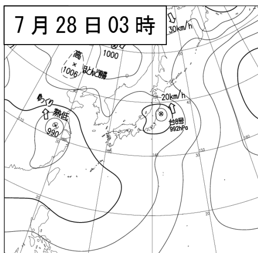
(3) 地上天気図及び気象衛星赤外面像 7月28日03時～29日15時：6時間毎
