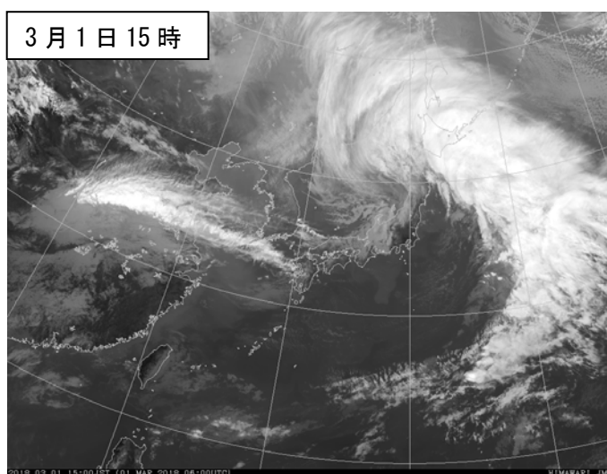
衛星画像（赤外）
