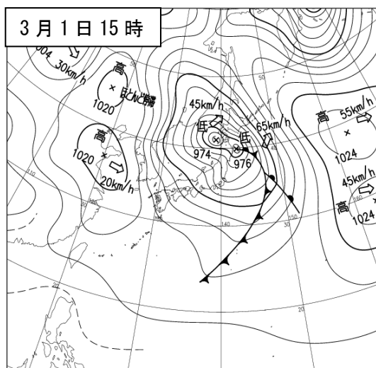
地上天気図
