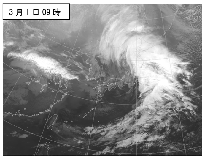
衛星画像 (赤外)
