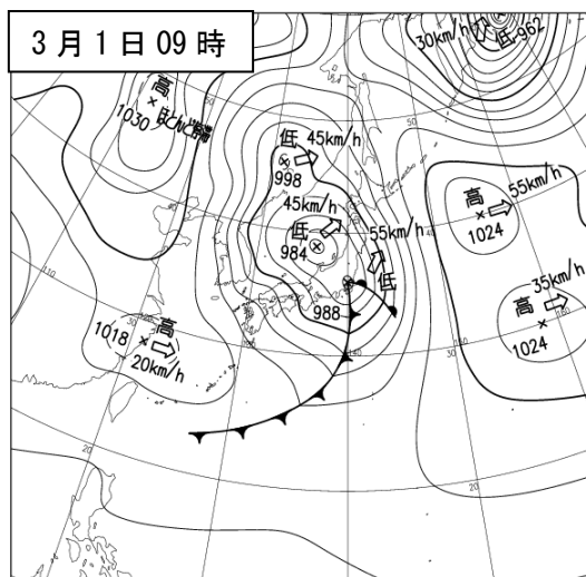
地上天気図
