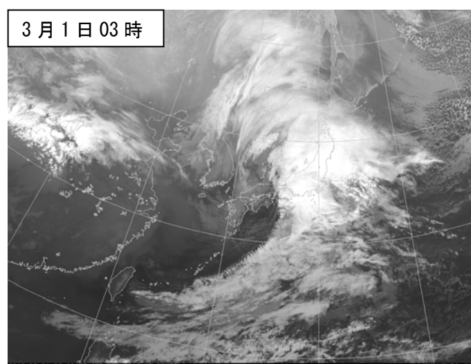
衛星画像 (赤外)
