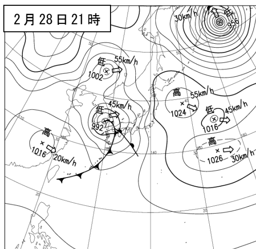
地上天気図
