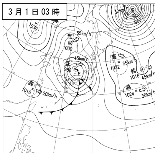
地上天気図
