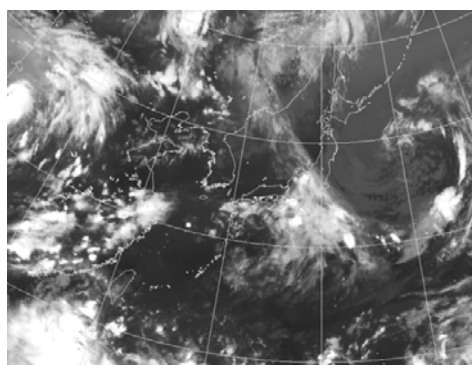
気象衛星赤外画像 (7月20日21時)
