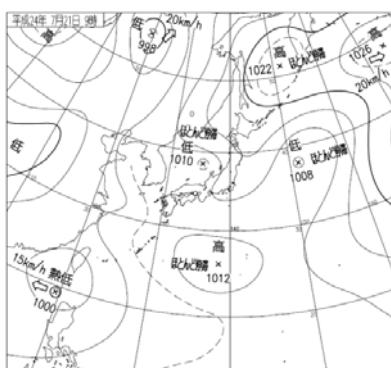
地上天気図 (7月21日09時)
