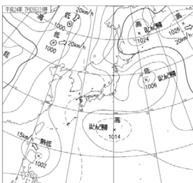
地上天気図 (7月20日21時)
