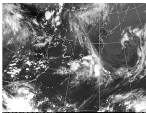
気象衛星赤外画像 (7月20日15時)
