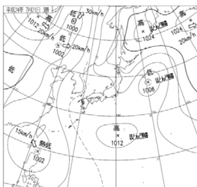
地上天気図 (7月21日03時)
