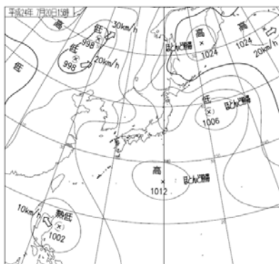
地上天気図 (7月20日15時)
