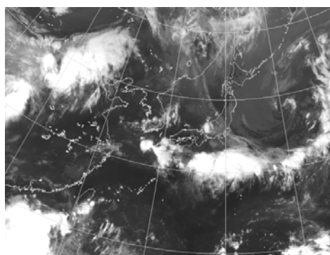
気象衛星赤外画像 (7月21日09時)
