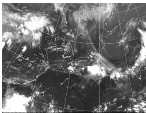
気象衛星赤外画像 (7月21日03時)
