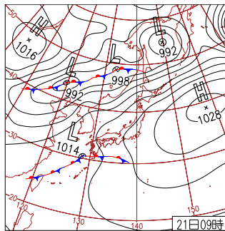
21日（木）函館市でサクラ開花 前線や発達する低気圧の影響により午前中西日本中心の雨は夜には東北南部まで広がる。北海道は概ね晴れて、最高気温が最も暑い時期を上回る所も。函館市でサクラ開花。
