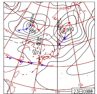
23日（土）札幌市でサクラ開花 オホーツク海の低気圧や前線の影響で北日本では風が強く、東北で雨。日本の南の前線の影響で、九州～四国を中心に雨。静岡県磐田など3地点で4月の最高気温の1位を記録。
