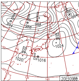
20日（水）青森市でサクラ満開 日本の東と東シナ海の高気圧に覆われ晴れた所多く、西日本内陸は夏日。北海道では最高気温6～7月中旬並の所も。関東では湿った空気の影響で曇りや雨。札幌市などウメ開花。
