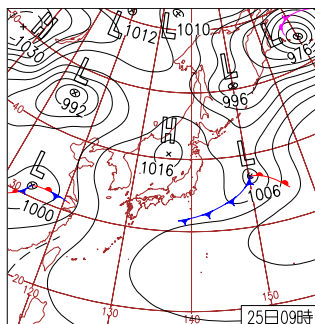
25日（月）北海道各地サクラ満開 高気圧に覆われ広く晴れ。気圧の谷の影響で沖縄～九州・四国は曇りや雨の所も。大分県日田4月1位の最高気温31.5℃。函館市、札幌市、帯広市サクラ満開。室蘭市サクラ開花。
