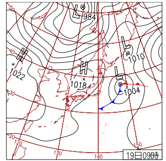
19日（火）茨城県で震度5弱 日本の東の低気圧や気圧の谷の影響で南西諸島や九州～関東の太平洋側では雲が多く所々で雨。また北陸～東北の一部で雨の所も。その他は日本海の高気圧に覆われ晴れ。
