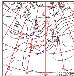
22日（金）関東甲信で気温上がる 三陸沖と沿海州の低気圧や前線の影響により東日本～北海道で雨や曇り。次第に高気圧に覆われ西日本～東日本太平洋側は晴れて7月並の最高気温の所も。帯広市でサクラ開花。
