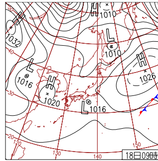
18日（月）東日本中心に雨 北日本の一部で午前中晴れた他は、日本付近は気圧の谷で、全般に曇り。東海道沖の低気圧の影響で東日本を中心に雨。西日本や北日本の所々でも雨。盛岡市でサクラ満開。
