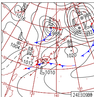
24日（日）南岸に前線停滞 南岸の前線上を低気圧が東進。沖縄・奄美や西～東日本で雨や曇り。1時間降水量は鹿児島県さつま柏原50.5mm、川内46.5mmで4月の1位更新。北日本は概ね晴れ。
