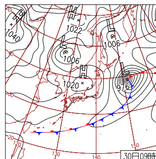
30日（土）北日本は花冷え 低気圧が日本の東へ去り南西諸島は前線の影響で曇りや雨、他は高気圧に覆われ概ね晴れ。東北で未明まで雪。北日本は最低気温3月中下旬並の所も。室蘭市、網走市サクラ満開。
