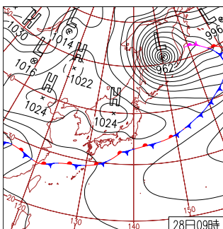
28日（木）旭川市でサクラ満開 高気圧に覆われて晴れた所が多かった。日本の南の前線の影響で西～東日本太平洋側で午前を中心に曇り。奄美や九州～四国の一部で雨。沖縄県の8地点と大分県日田で真夏日。
