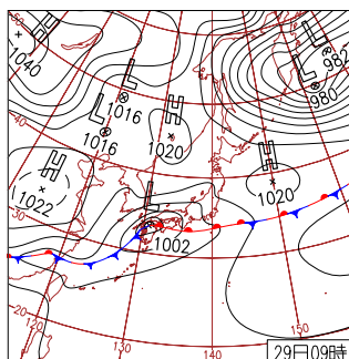
29日（金）沖縄県で真夏日多数 九州の低気圧の影響で九州～東北は所々で雨。北海道や沖縄県では晴れた所も。晴れて南西からの暖かい風が吹いた沖縄県では真夏日多数。4月の最高気温の記録更新の所も。
