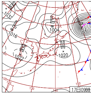
17日（日）東海～関東で雨 高気圧に緩やかに覆われ広い範囲で晴れたが、東海～関東は湿った空気や気圧の谷の影響で雨や曇りとなり、最高気温が2月下旬並の所も。北海道は低気圧の接近で雨や曇りの所も。
