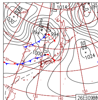
26日（火）旭川市でサクラ開花 中国大陸と日本海の前線を伴った低気圧が発達しながら東進。日本の東の高気圧の縁を沿う南からの湿った空気の影響で全国的に雨や曇り。広い範囲で1時間降水量4月1位更新。
