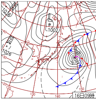
16日（土）次第に全国的に晴れ 午前中は東日本～東北は前線や湿った空気の影響により曇りや雨となったが、次第に高気圧に覆われて全国的に晴れ。青森市でサクラ開花。秋田市でサクラ満開。
