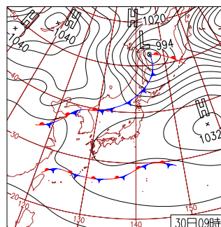
30日(水)西～東日本サクラ満開 前線の影響で南西諸島や九州では雲が多く所々雨。北海道でも寒冷前線の通過で雨や雪。その他は概ね晴れ。西～東日本の多くでサクラ満開。金沢市と水戸市ではサクラ開花。
