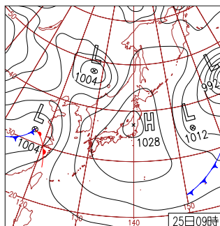
25日(金)福島県で震度4 高気圧は夜には日本の東へ。黄海に前線を伴った低気圧があって北東進。西～北日本は概ね晴れ。熊本県八代の最大瞬間風速23.6m/sは3月1位。奈良市など4地点でサクラ開花。
