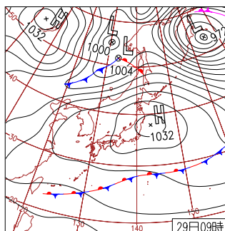
29日(火)広島市などでサクラ満開 本州付近は高気圧に覆われるが沖縄～東日本は前線や気圧の谷の影響で曇り。奄美と西～東日本太平洋側の所々で雨。北日本は概ね晴れ。長崎市、広島市、和歌山市でサクラ満開。
