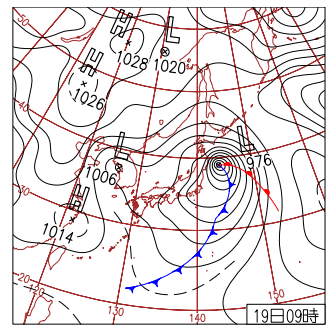
19日(土)北日本で大荒れ 三陸沖の低気圧の影響で北日本太平洋側は暴風雪や大雪。西～東日本も寒気の影響で荒れた天気。北海道えりも岬は最大風速33.8m/sで3月1位。高知市、佐賀市でサクラ開花。
