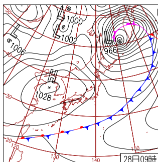
28日(月)各地でサクラ満開 沖縄～九州南部は前線や湿った空気の影響で雨。北日本ははじめ雨や雪が降ったが次第に高気圧に覆われて晴れ。その他は晴れや曇り。松山市や横浜市など7地点でサクラ満開。
