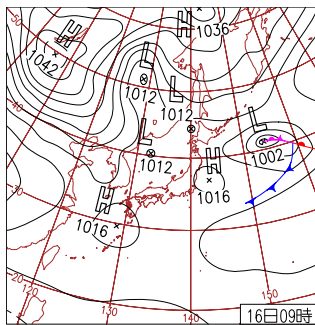
16日(水)福島県宮城県で震度6強 九州付近と関東の東海上の高気圧に覆われ、南西諸島～東日本は晴れて気温上昇。北海道付近の低気圧の影響で北日本では曇りとなり、所々で雪や雨を観測。
