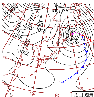
20日(日)東京などでサクラ開花 北日本は冬型の気圧配置で、西日本は中国大陸からの高気圧に覆れる。日本海側は雲が多く所々で雪や雨。太平洋側は概ね晴れ。鹿児島市、熊本市、東京でサクラ開花。
