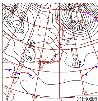
21日(月)各地でサクラ開花 北日本は冬型の気圧配置で北陸～北日本日本海側は雪や雨。東シナ海の前線の影響で南西諸島～西日本は次第に雨。その他は概ね晴れ。広島市や横浜市など6地点でサクラ開花。
