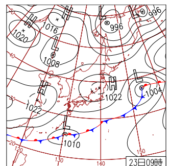
23日(水)西から次第に雨 沖縄～西日本は雨。東日本も次第に雨や雪。北日本は日中晴れたが次第に曇り、夜は雪の所も。東日本～東北の最低気温は最も寒い時期を下回る。大分市と大阪市でサクラ開花。
