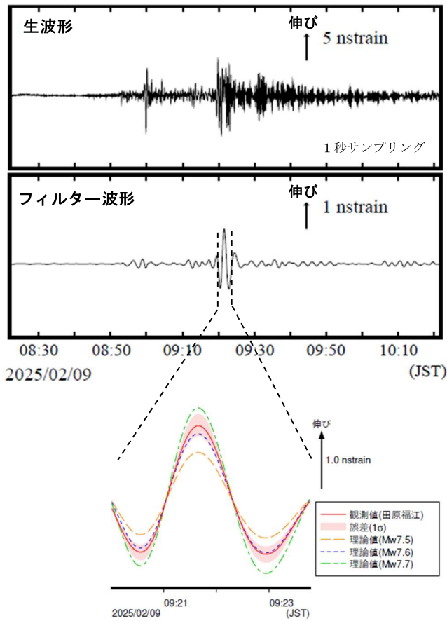
田原福江観測点で観測された体積ひずみ波形
