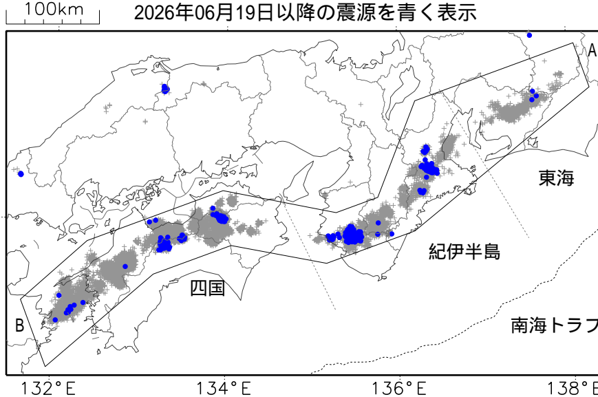
震央分布図（2025年06月26日～2026年06月25日：過去1年間、M全て、深さ全て）
