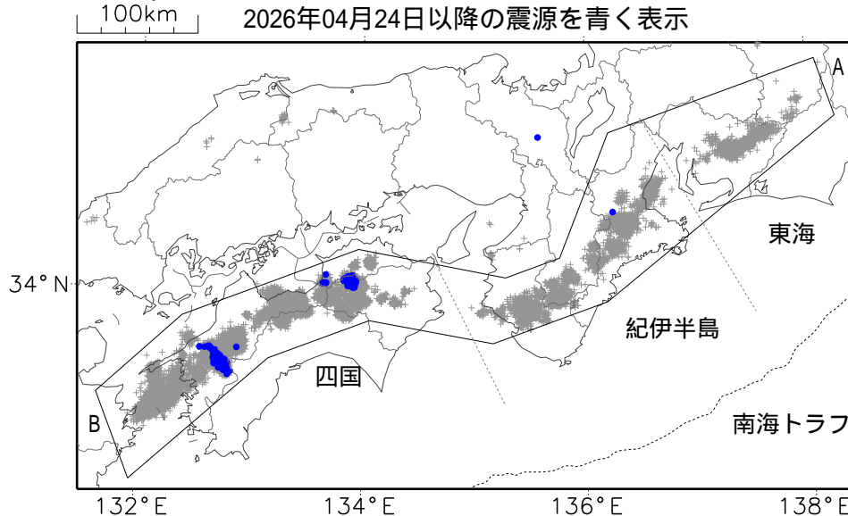
震央分布図（2025年05月01日～2026年04月30日：過去1年間、M全て、深さ全て）
