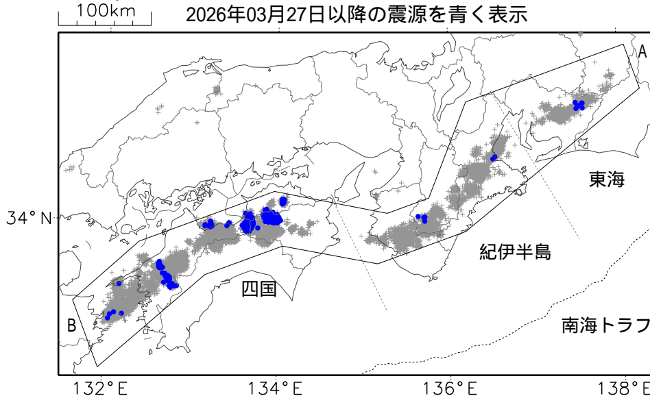
震央分布図（2025年04月03日～2026年04月02日：過去1年間、M全て、深さ全て）
