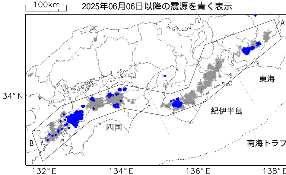
震央分布図（2024年06月13日～2025年06月12日：過去1年間、M全て、深さ全て）
