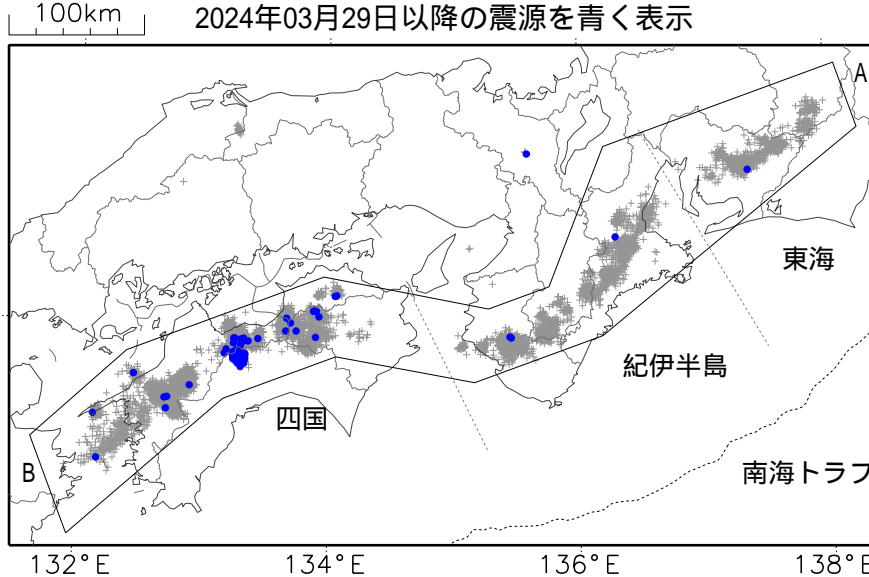
震央分布図（2023年04月05日～2024年04月04日：過去1年間、M全て、深さ全て）
