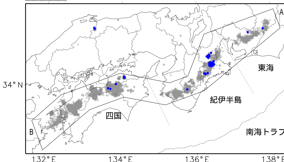
震央分布図（2023年03月15日～2024年03月14日：過去1年間、M全て、深さ全て） 2024年03月08日以降の震源を青く表示
