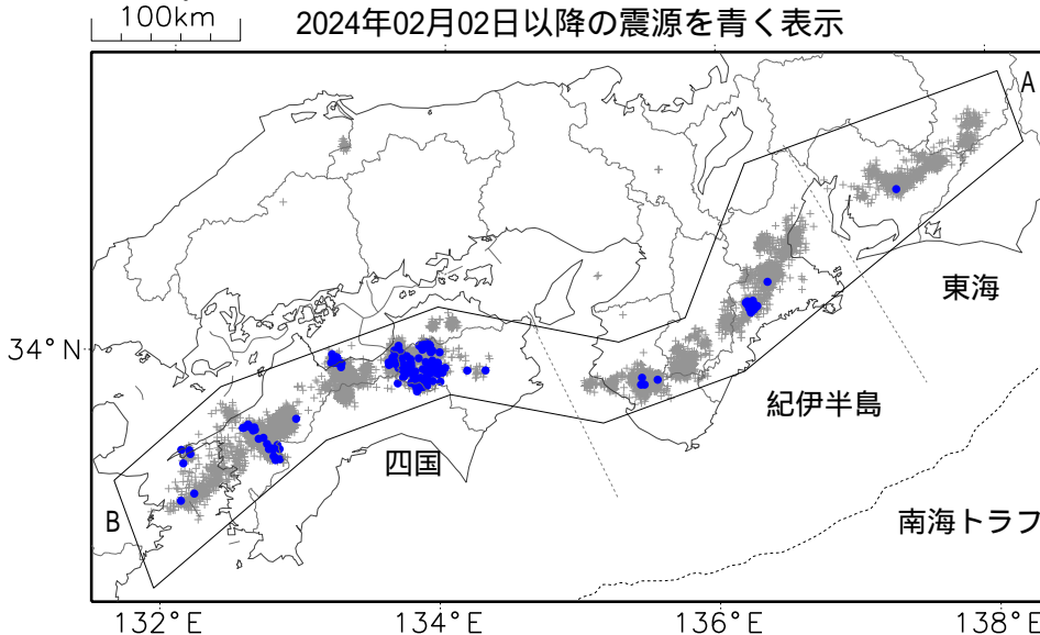
震央分布図（2023年02月09日～2024年02月08日：過去1年間、M全て、深さ全て）
