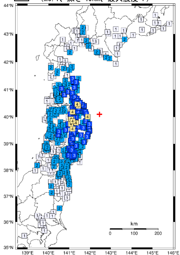
図4 震度分布図
