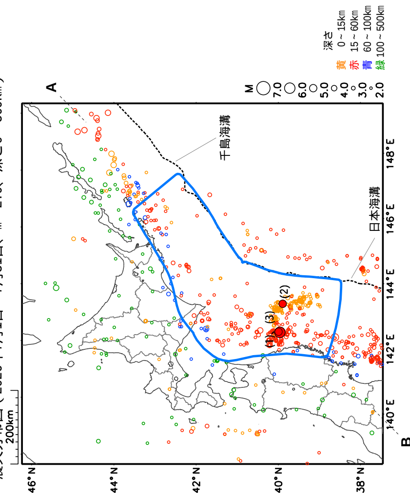
震央分布図（2026年7月1日～7月31日、M 2.0、深さ0～500km）
