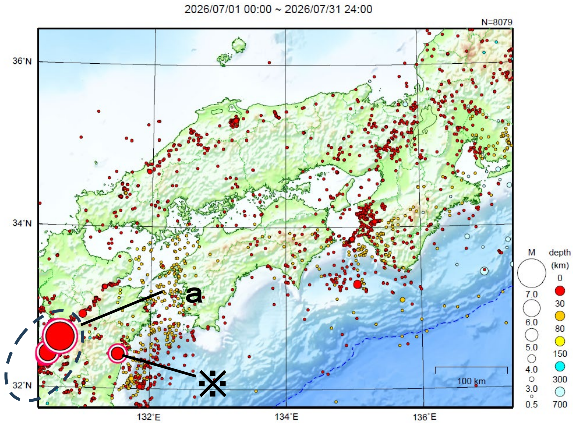
図 8 近畿・中国・四国地方の震央分布図（2026 年 7 月 1 日～7 月 31 日、M≥0.5）
