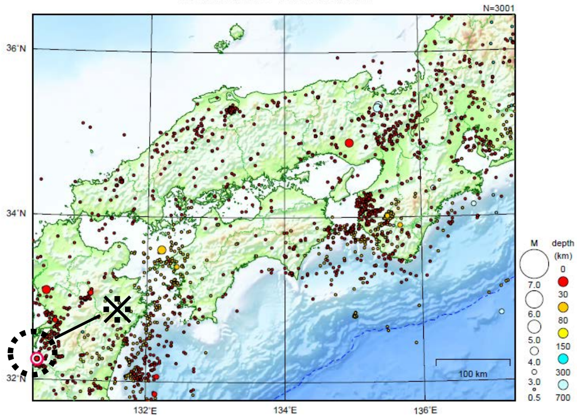
図8 近畿・中国・四国地方の震央分布図（2026年3月1日～3月31日、 M \geq 0.5 ）
