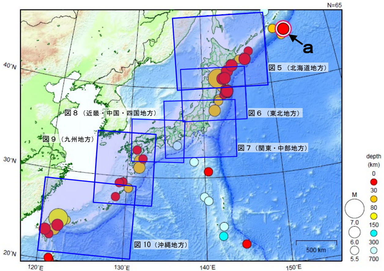
図11 日本周辺で発生した主な地震の震央分布図（2025年1月1日～12月31日、M≥5.5）
