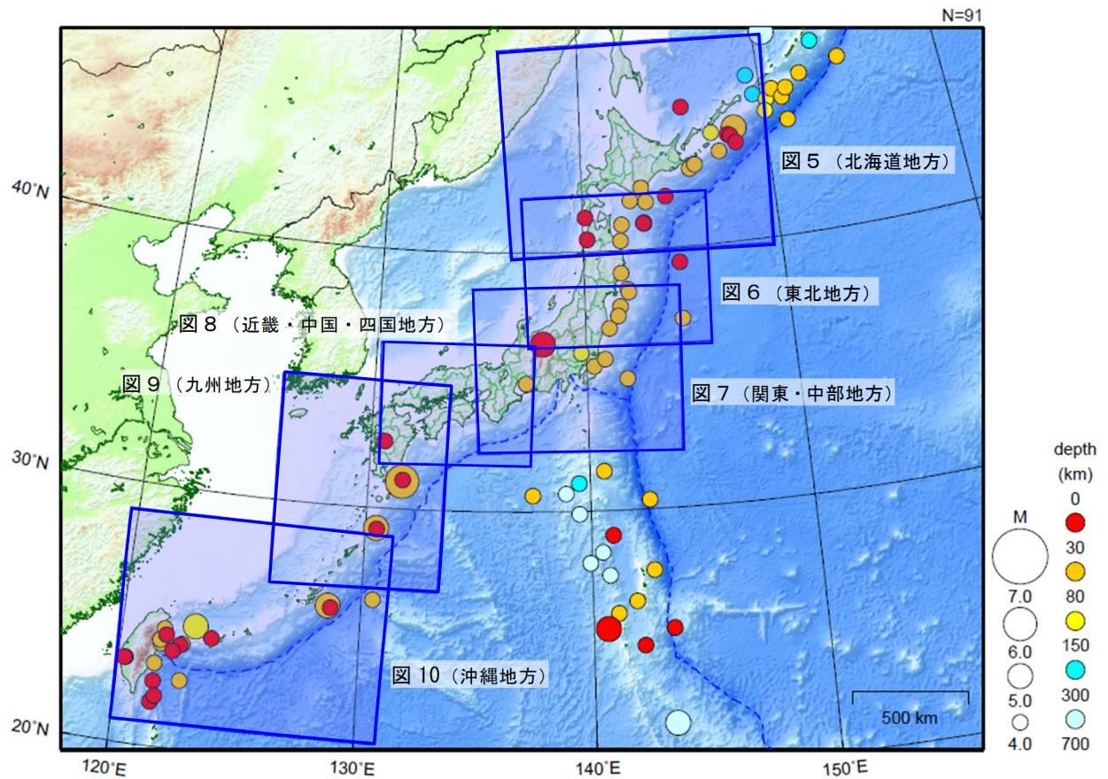
図11 日本周辺で発生した主な地震の震央分布図（2025年4月1日～4月30日、 M \geq 4.0 ）
