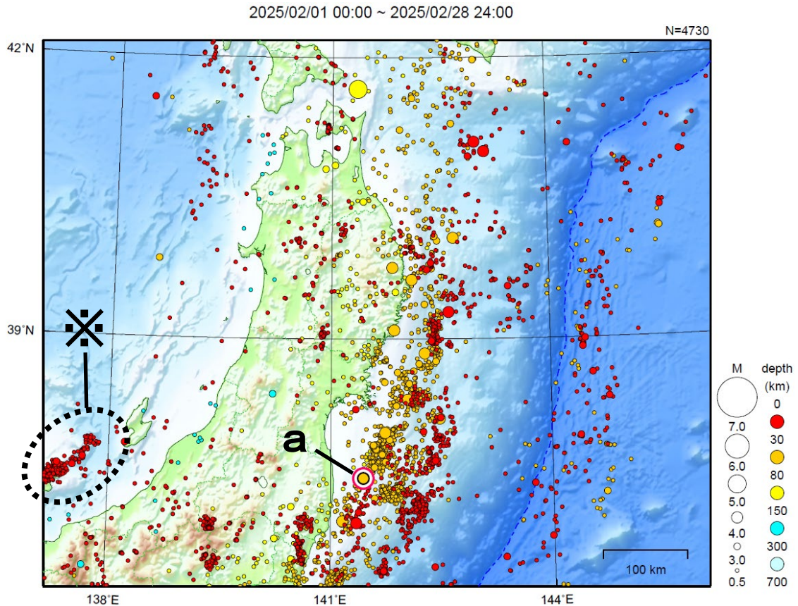
図 6 東北地方の震央分布図（2025 年 2 月 1 日～2 月 28 日、 M \geq 0.5 ）
