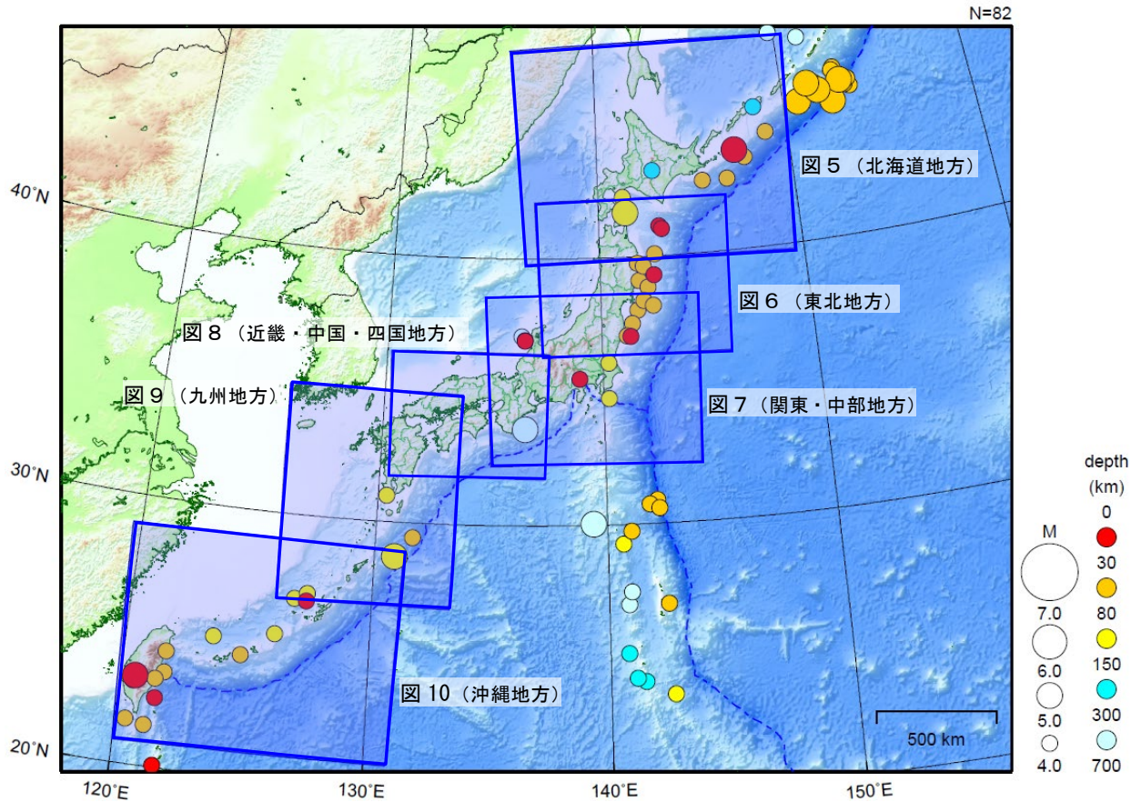
図11 日本周辺で発生した主な地震の震央分布図（2025年2月1日～2月28日、 M \geq 4.0 ）
