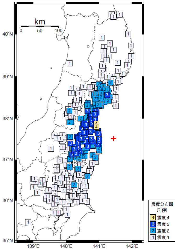
図4 震度分布図 (各図の左上の数字は表1、図2、図3の番号に対応する。赤の+印は震央を示す)
