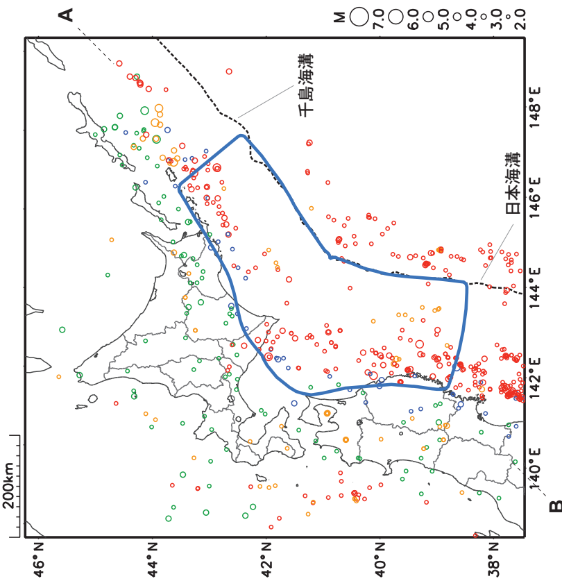
震央分布図 (2024年12月1日～12月31日、 M \geq 2.0 、深さ0～500km)
