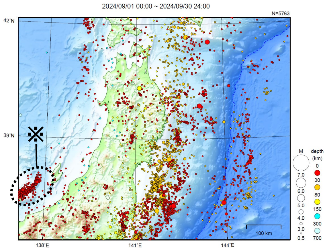
図6 東北地方の震央分布図（2024年9月1日～9月30日、 M \geq 0.5 ）
