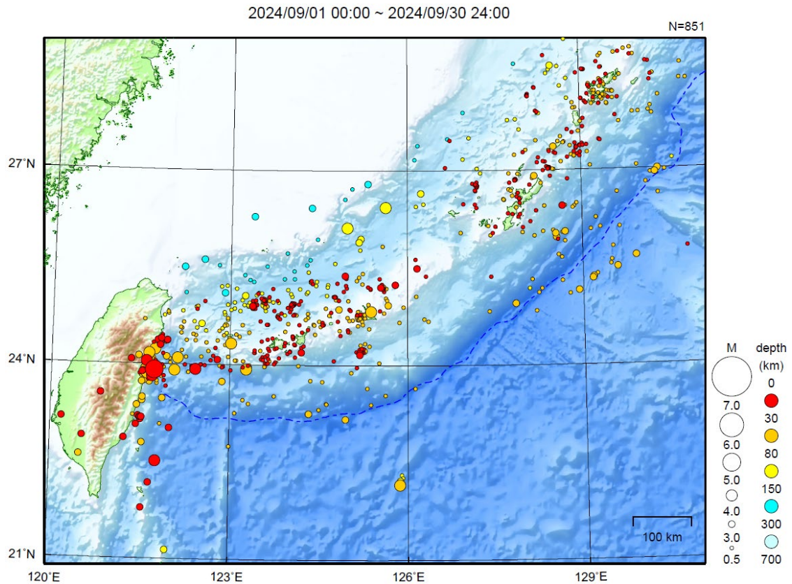
図 10 沖縄地方の震央分布図（2024 年 9 月 1 日～9 月 30 日、 M \geq 0.5 ）
