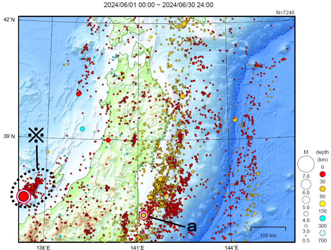
図6 東北地方の震央分布図（2024年6月1日～6月30日、 M \geq 0.5 ）
