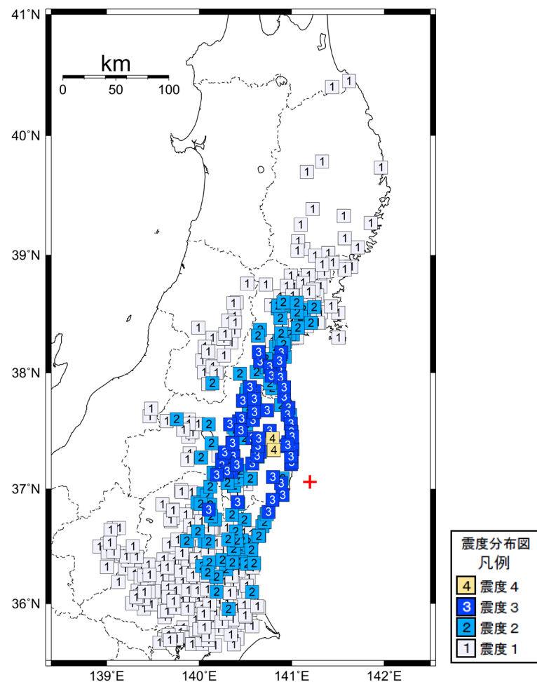
図4 震度分布図（続き） （各図の左上の数字は表1、図2、図3の番号に対応する。赤の+印は震央を示す）
