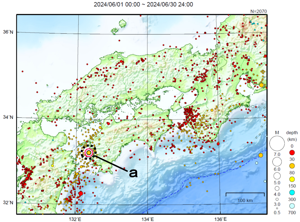
図 8 近畿・中国・四国地方の震央分布図（2024 年 6 月 1 日～6 月 30 日、 M \geq 0.5 ）
