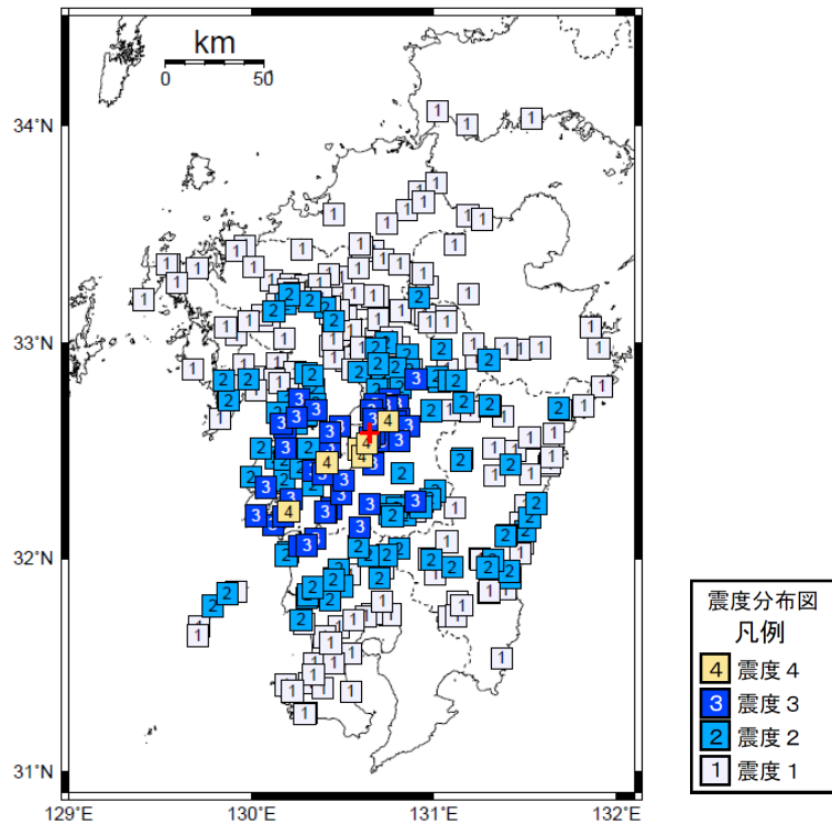
図4 震度分布図
