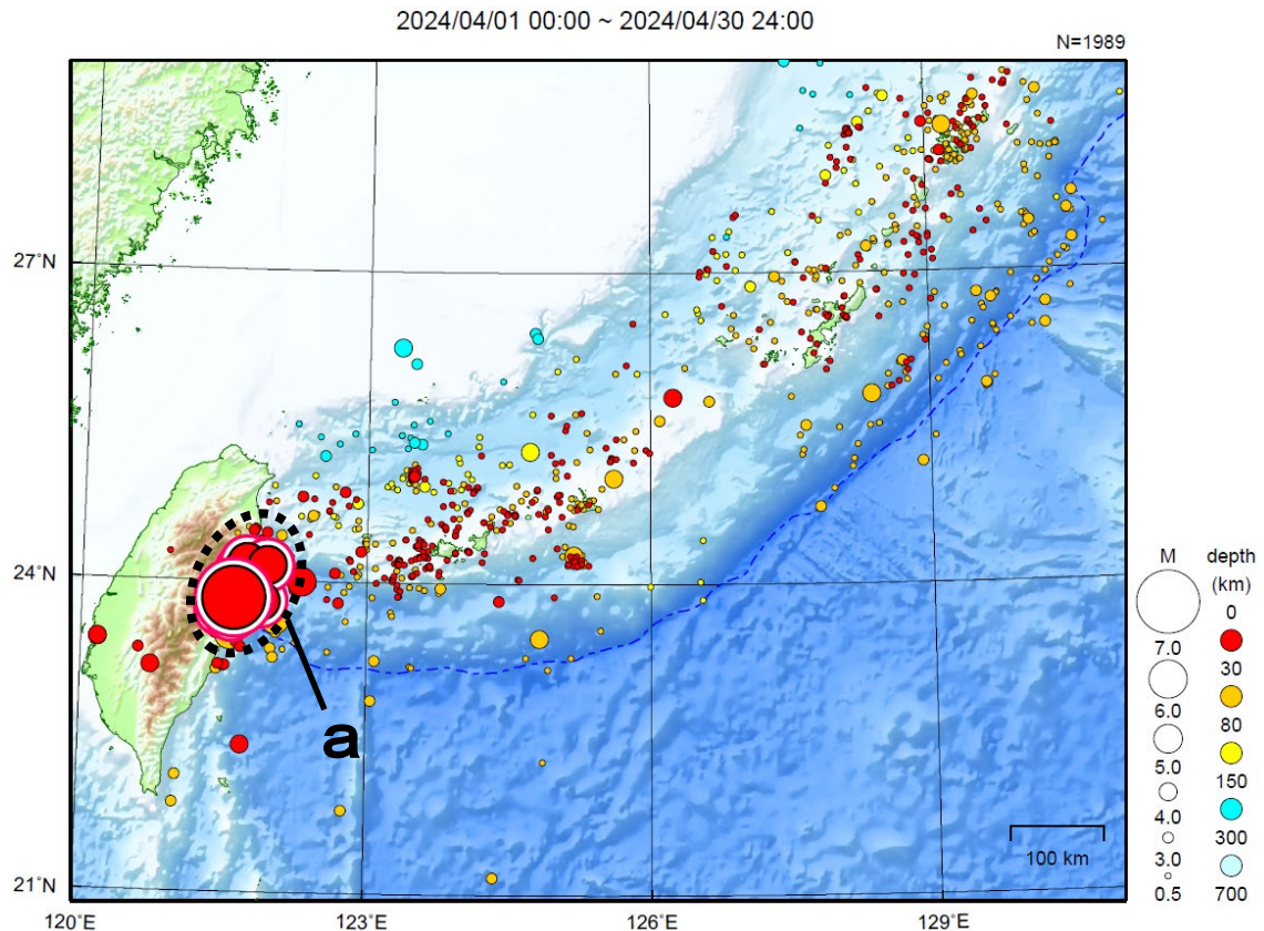
図 10 沖縄地方の震央分布図（2024 年 4 月 1 日～4 月 30 日、 M \geq 0.5 ）
