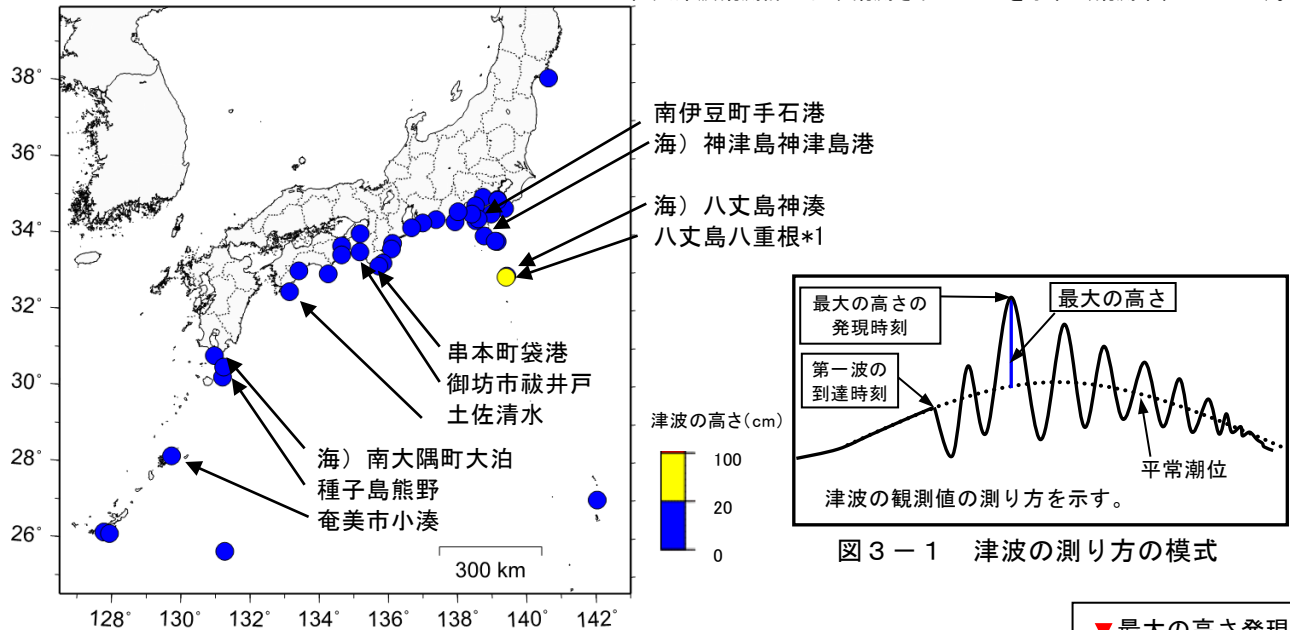
図3-2 津波を観測した地点
