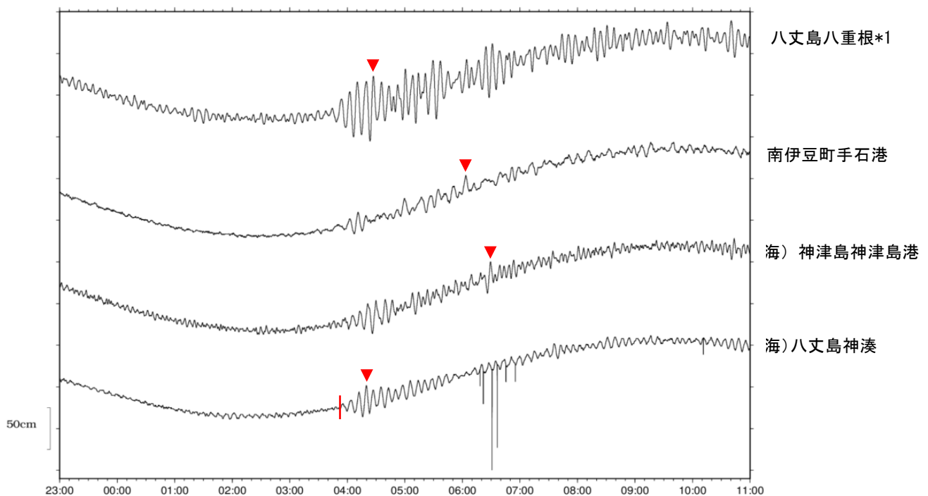
図3-3-1 主な津波波形（2023年12月2日23時から3日11時まで）
