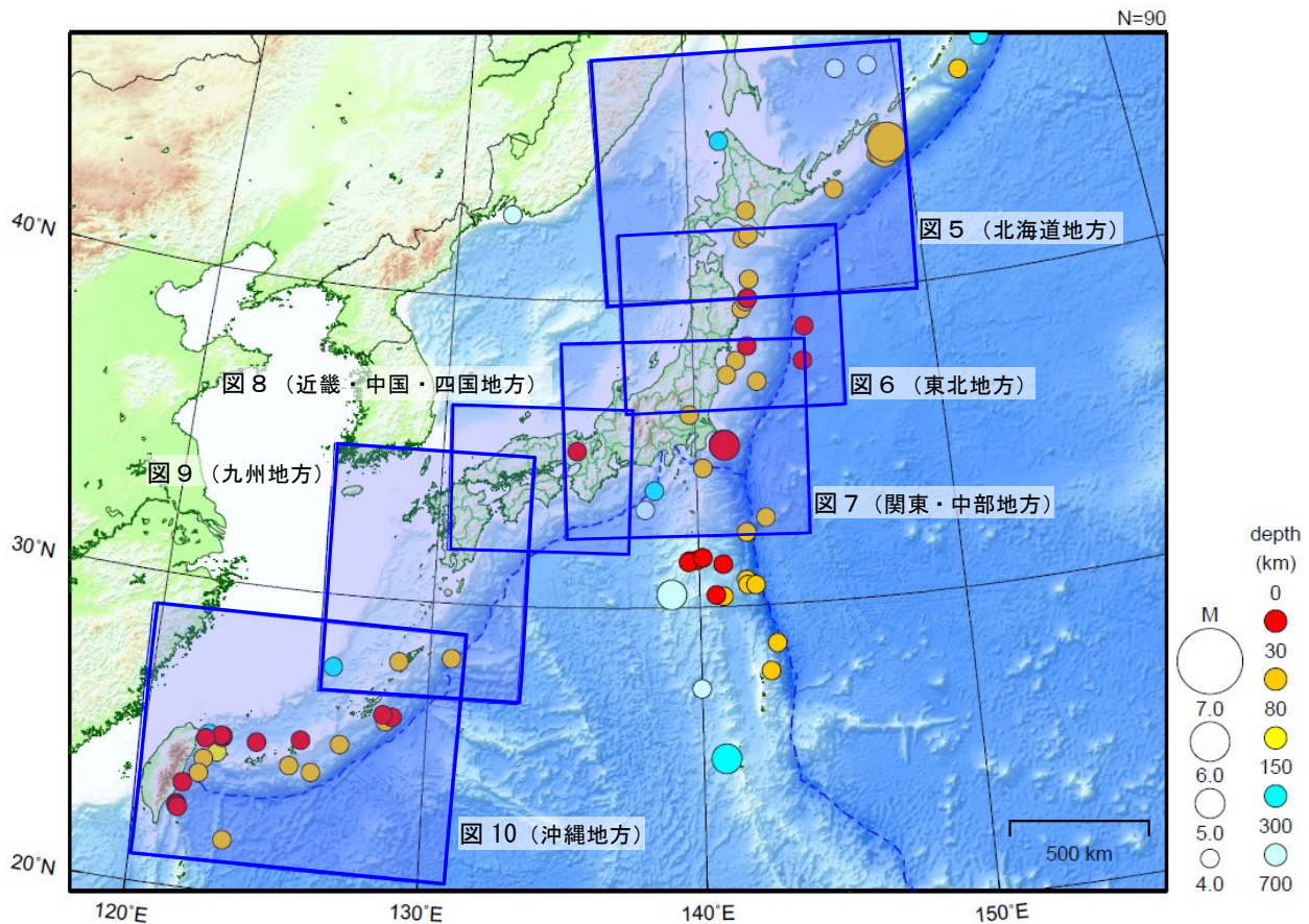
図10 日本周辺で発生した主な地震の震央分布図 (2023年12月1日~12月31日、 M \geq 4.0 )
