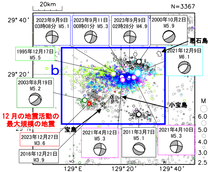
震央分布図
