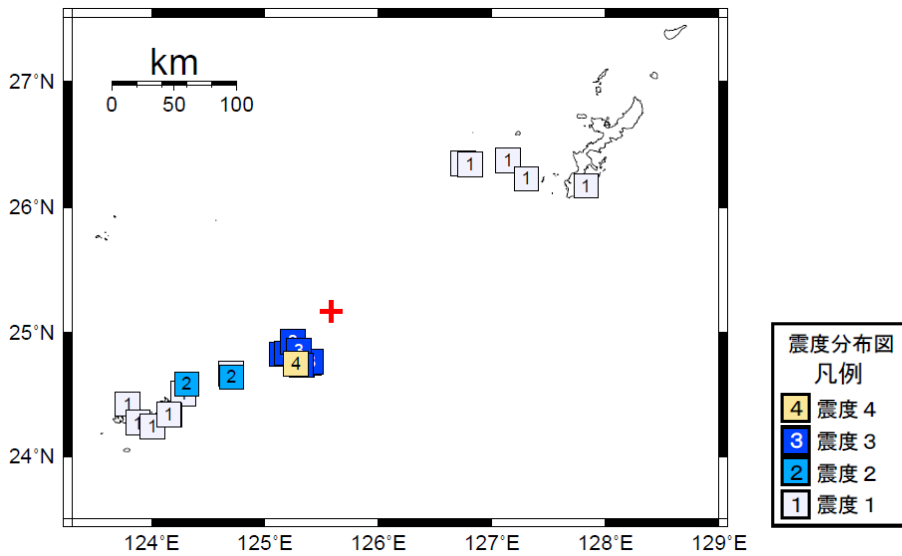
図4 震度分布図
