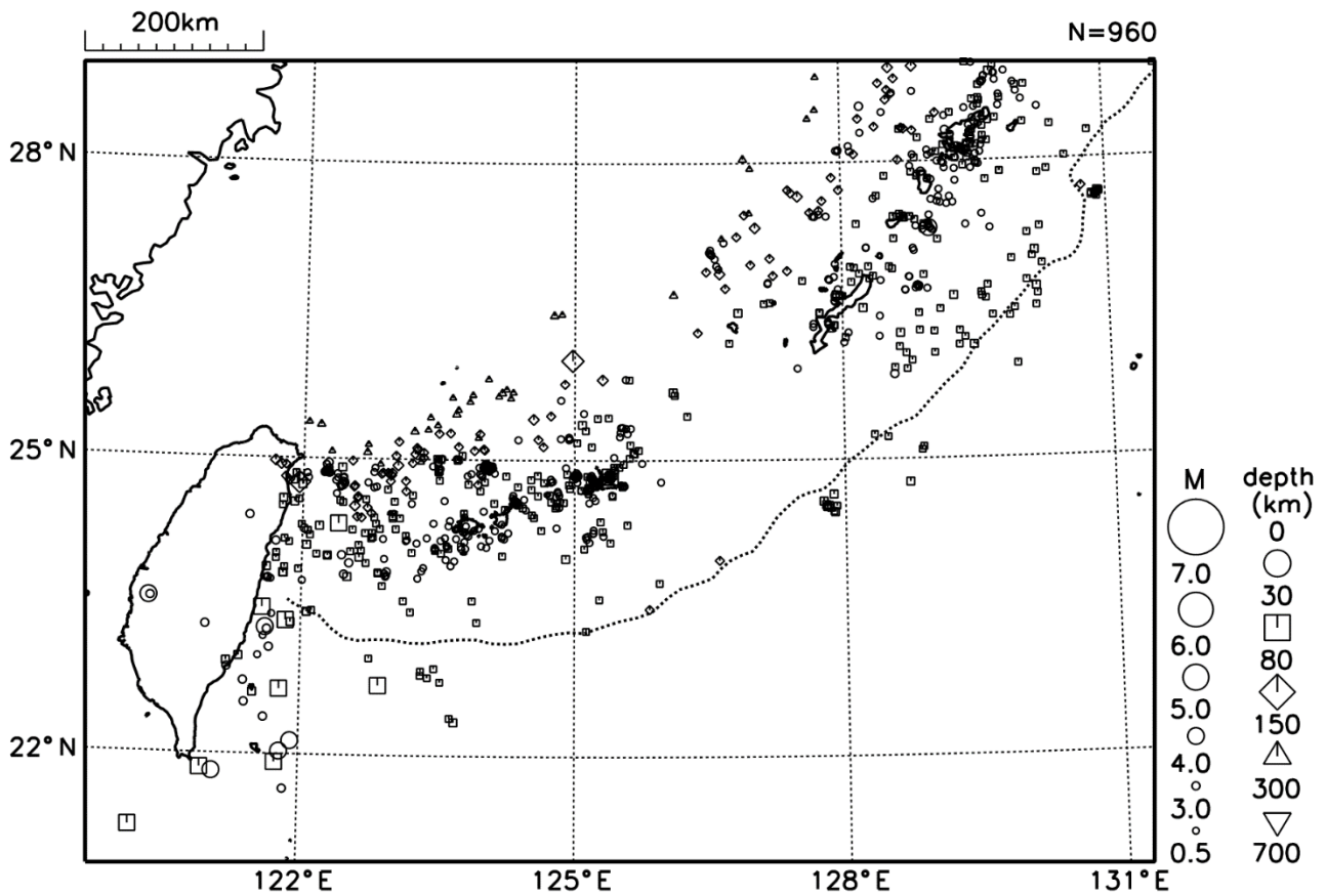
図10 沖縄地方の震央分布図（2023年8月1日～8月31日、 M \geq 0.5 ）
