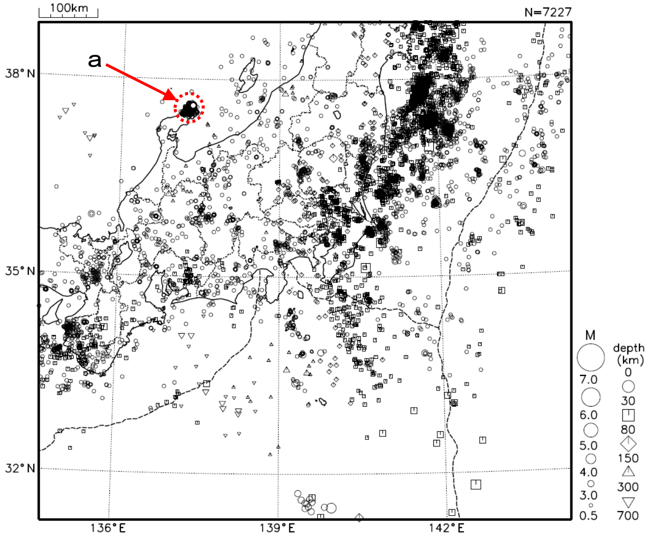
図7 関東・中部地方の震央分布図（2023年8月1日～8月31日、 M \geq 0.5 ）
