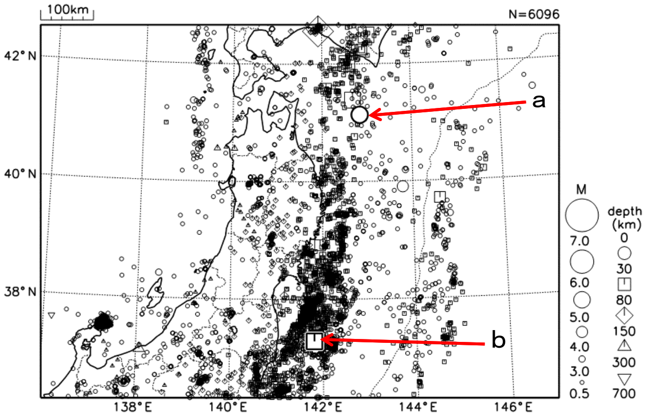
図6 東北地方の震央分布図（2023年6月1日～6月30日、 M \geq 0.5 ）
