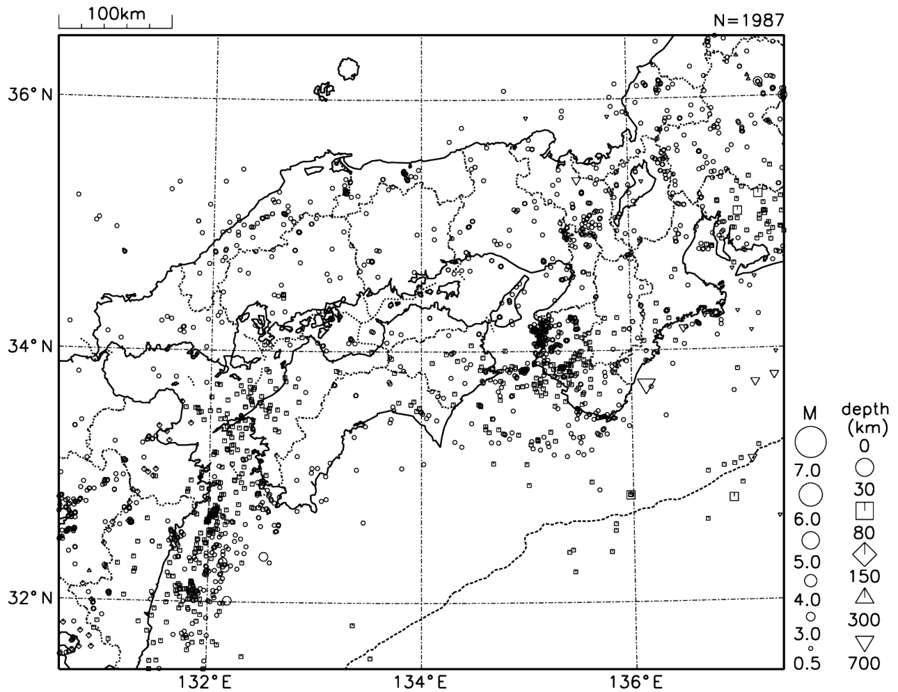
図8 近畿・中国・四国地方の震央分布図（2023年6月1日～6月30日、 M \geq 0.5 ）
