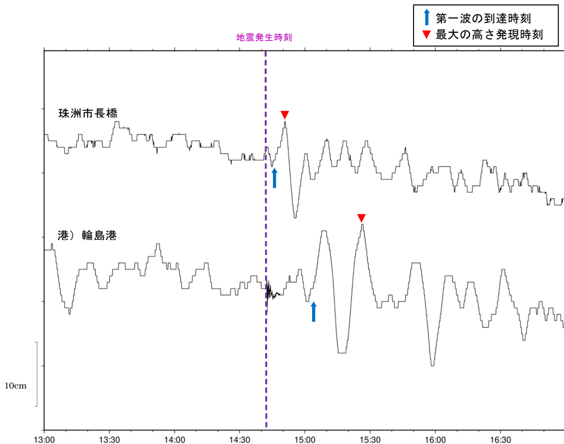
図6－3 津波波形
