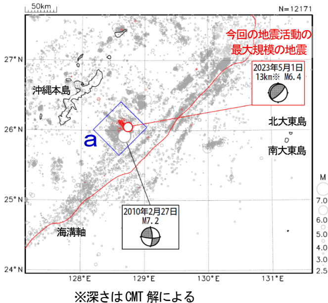
震央分布図 (2000年7月1日～2023年5月7日、 深さ0km～90km、 M \geq 2.5 ) 4月27日以降の地震を赤色で表示 図中の発震機構はCMT解
