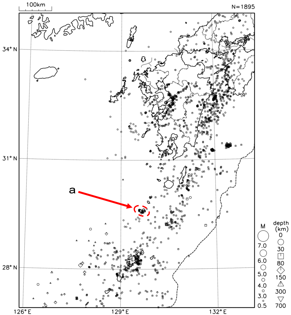
図9 九州地方の震央分布図（2022年9月1日～9月30日、M \geq 0.5）
