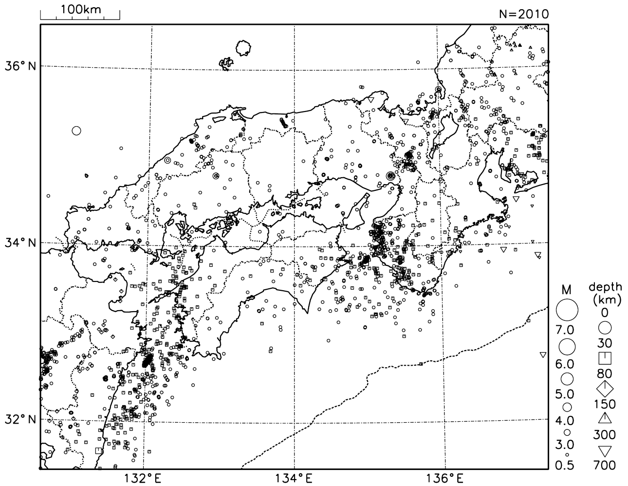
図8 近畿・中国・四国地方の震央分布図（2022年9月1日～9月30日、 M \geq 0.5 ）
