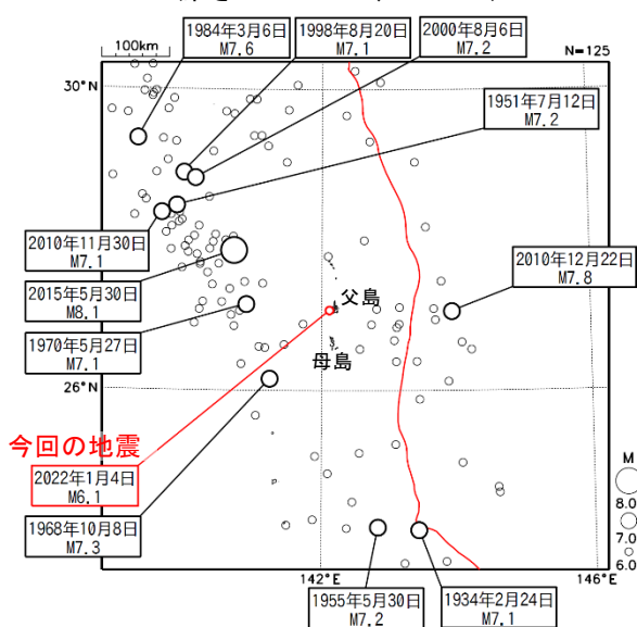
震央分布図
