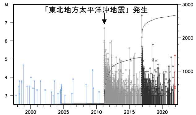
領域 b 内のM-T図及び回数積算図 (深さ0～40km)
