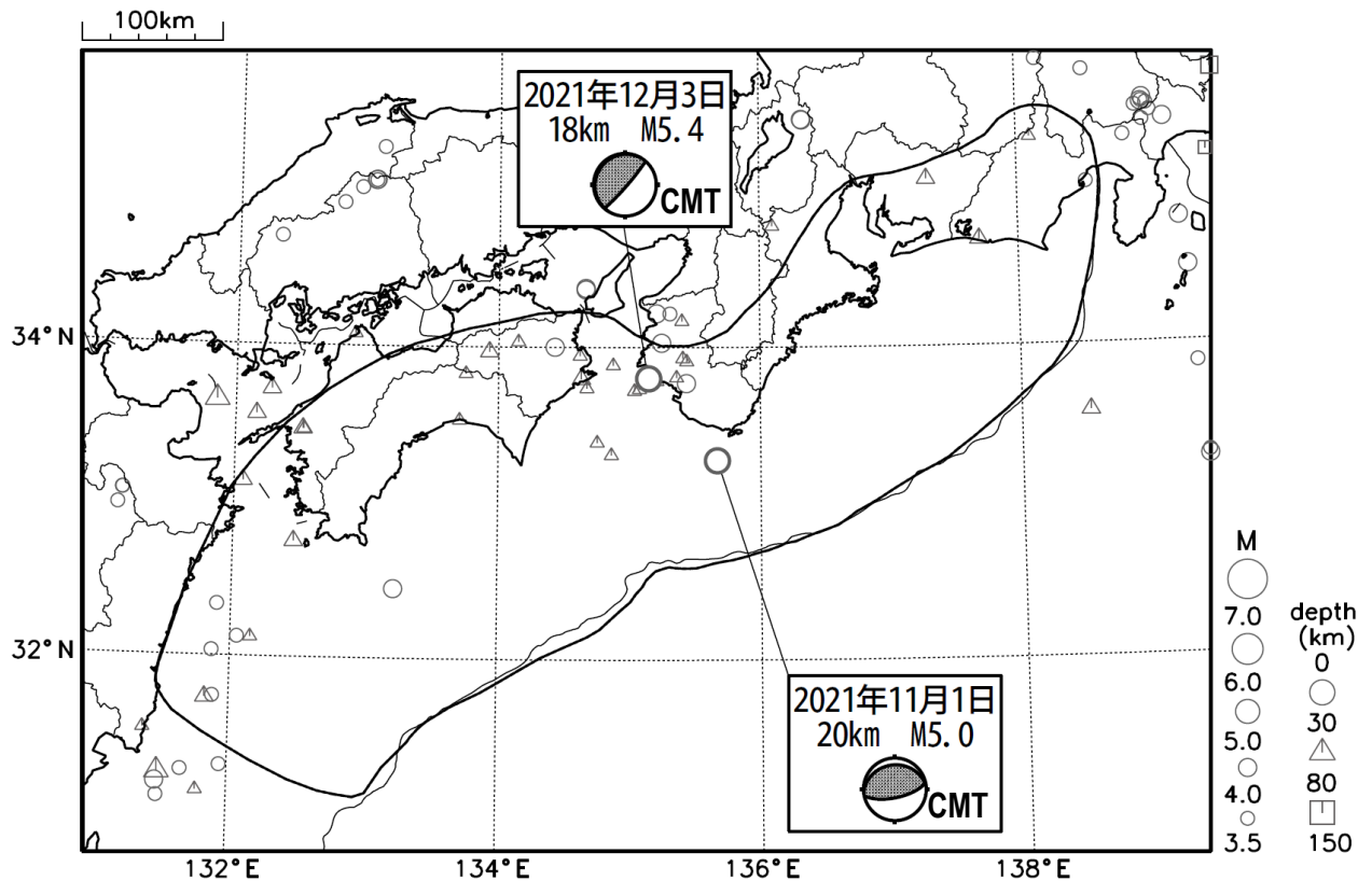
震央分布図（2021年1月1日～12月31日、深さ0～150km、 M \geq 3.5 ）
