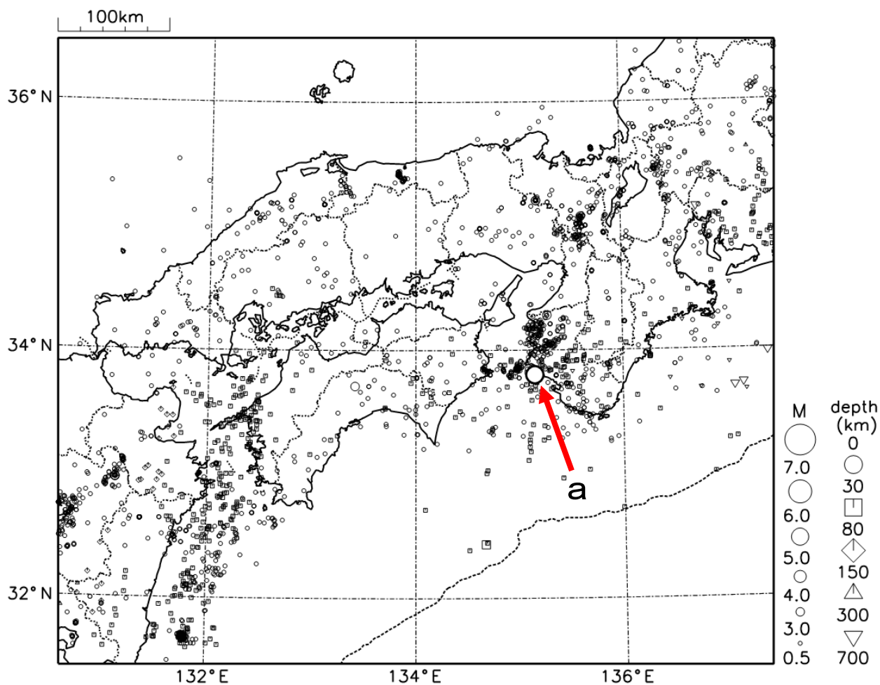
図8 近畿・中国・四国地方の震央分布図（2021年12月1日～12月31日、 M \geq 0.5 ）
