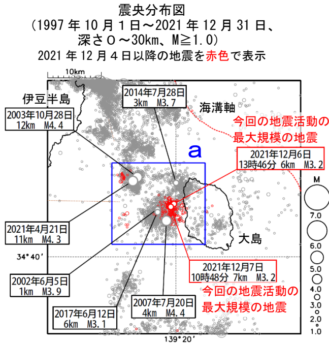
領域a内で発生した地震による 日別・震度別地震発生回数
