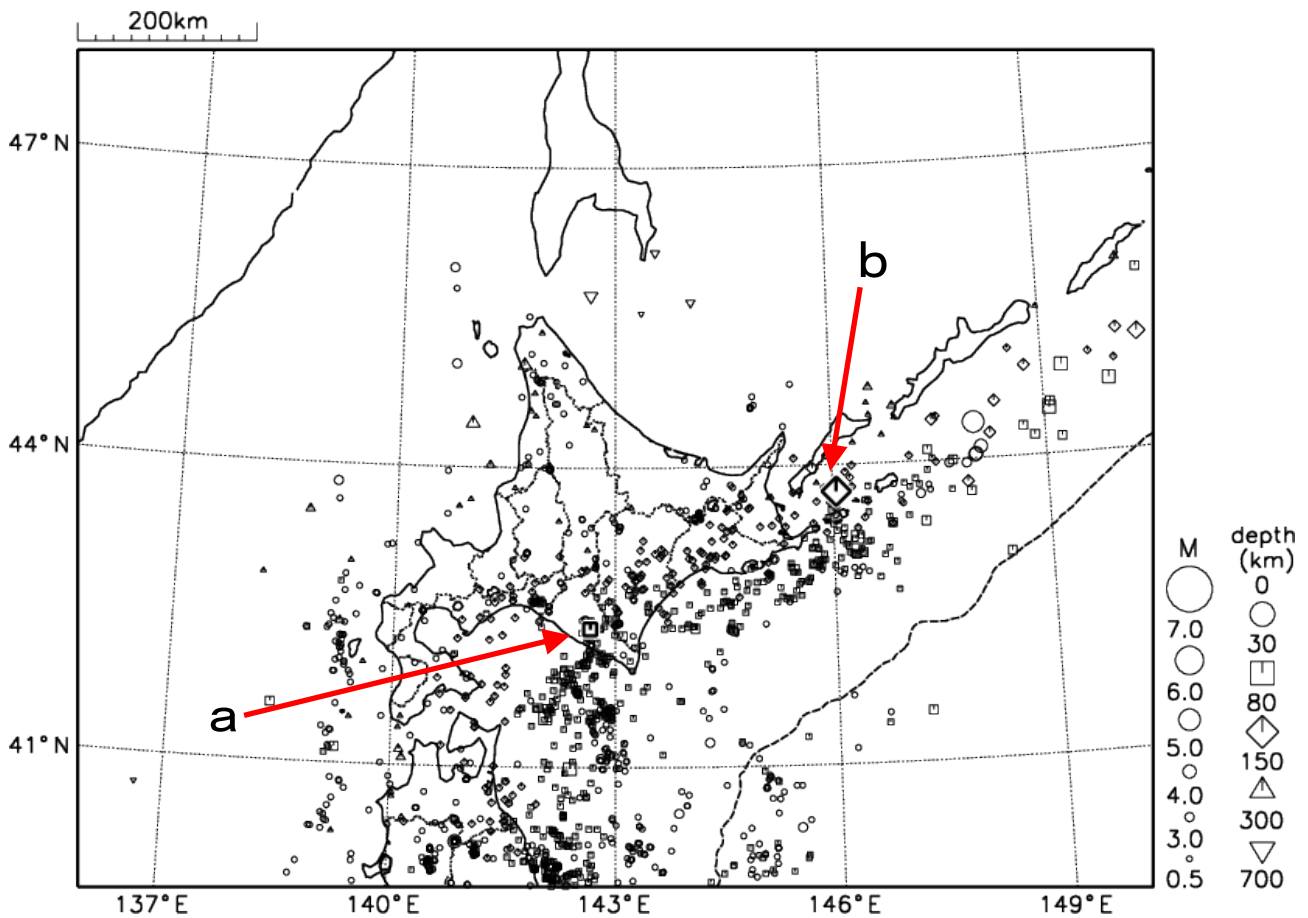
図5 北海道地方の震央分布図（2021年12月1日～12月31日、 M \geq 0.5 ）
